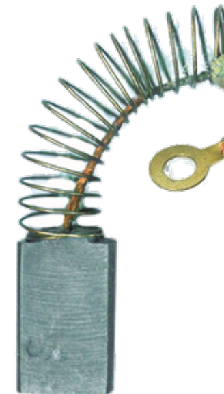
REF. 130 ROSCADORAS RIDGID 300 MOD. 535 8,7 x 19 x 31,9
