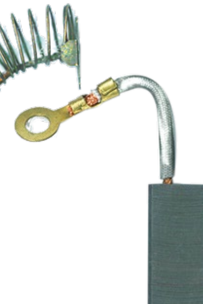
REF. E334 MOTOR MAQUINA ALGODON DE AZUCAR 7,9 x 16,3 x 32
