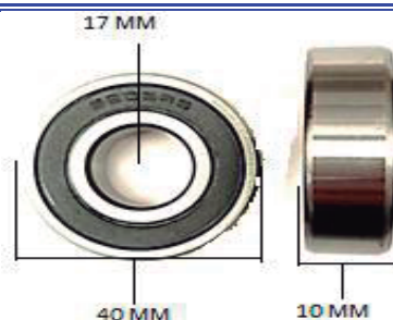
6203RS RODAMIENTO 17 X 40 X 10
