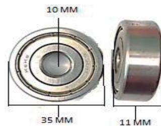
6300Z RODAMIENTO 10 X 35 X 11
