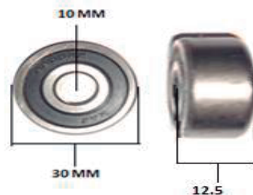
6200A O 87500 RS RODAMIENTO 10 X 30 X 12,5
