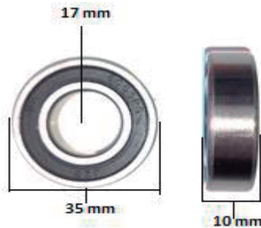
6003RS RODAMIENTO 17 X 35 X 10
