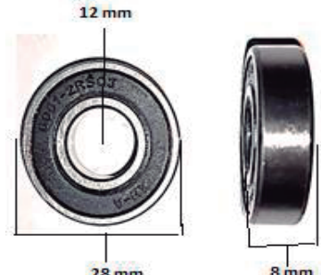
6001RS RODAMIENTO 12 X 28 X 8
