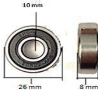
6000RS RODAMIENTO 10 X 26 X 8
