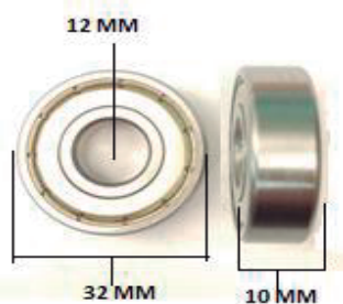
6201RS RODAMIENTO 12 X 32 X 10
