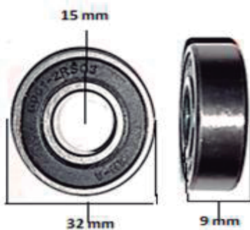
6002RS RODAMIENTO 15 X 32 X 9
