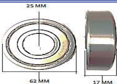
6305Z RODAMIENTO 25 X 62 X 17
