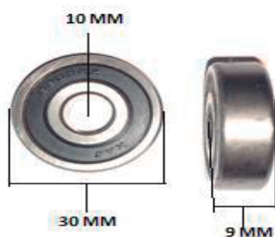
6200RS RODAMIENTO 10 X 30 X 9
