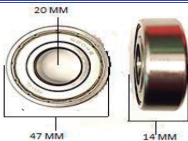
6204Z RODAMIENTO 20 X 47 X 14
