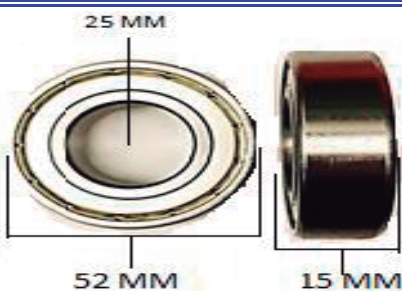
6205Z RODAMIENTO 25 X 52 X 15
