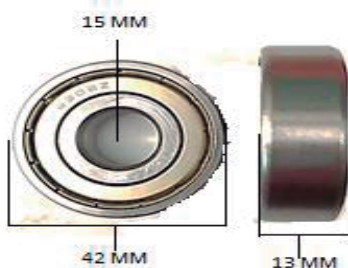
6302Z RODAMIENTO 15 X 42 X 13
