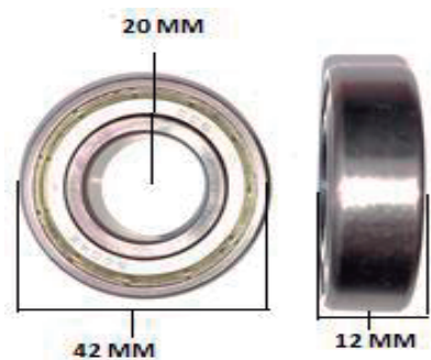
6004Z RODAMIENTO 20 X 42 X 12
