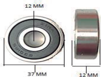
6301RS RODAMIENTO 12 X 37 X 12
