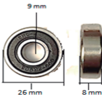
629RS RODAMIENTO 9 X 26 X 8
