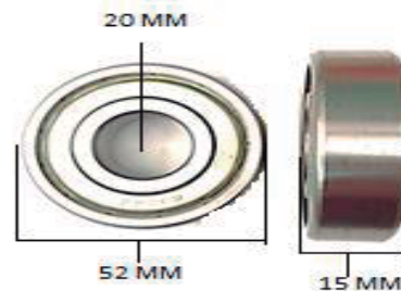
6304Z RODAMIENTO 20 X 52 X 15
