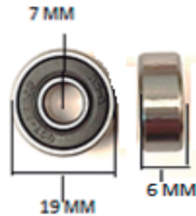
607RS RODAMIENTO 7 X 19 X 6
