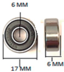
606RS RODAMIENTO 6 X 17 X 6
