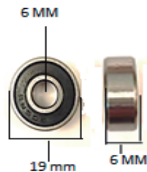
626RS RODAMIENTO 6 X 19 X 6
